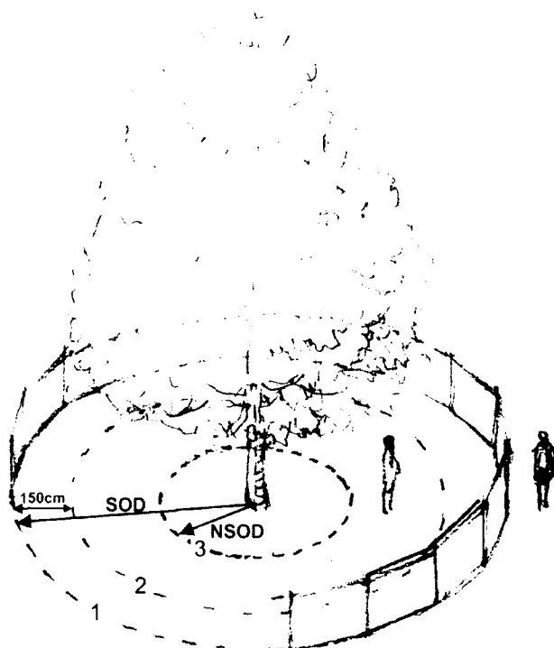
Ryc. 8. Standard zabezpieczenia drzewa na placu budowy - wygradzenie strefy ochrony drzewa. (Oprac. A. Kwaśniewska)
