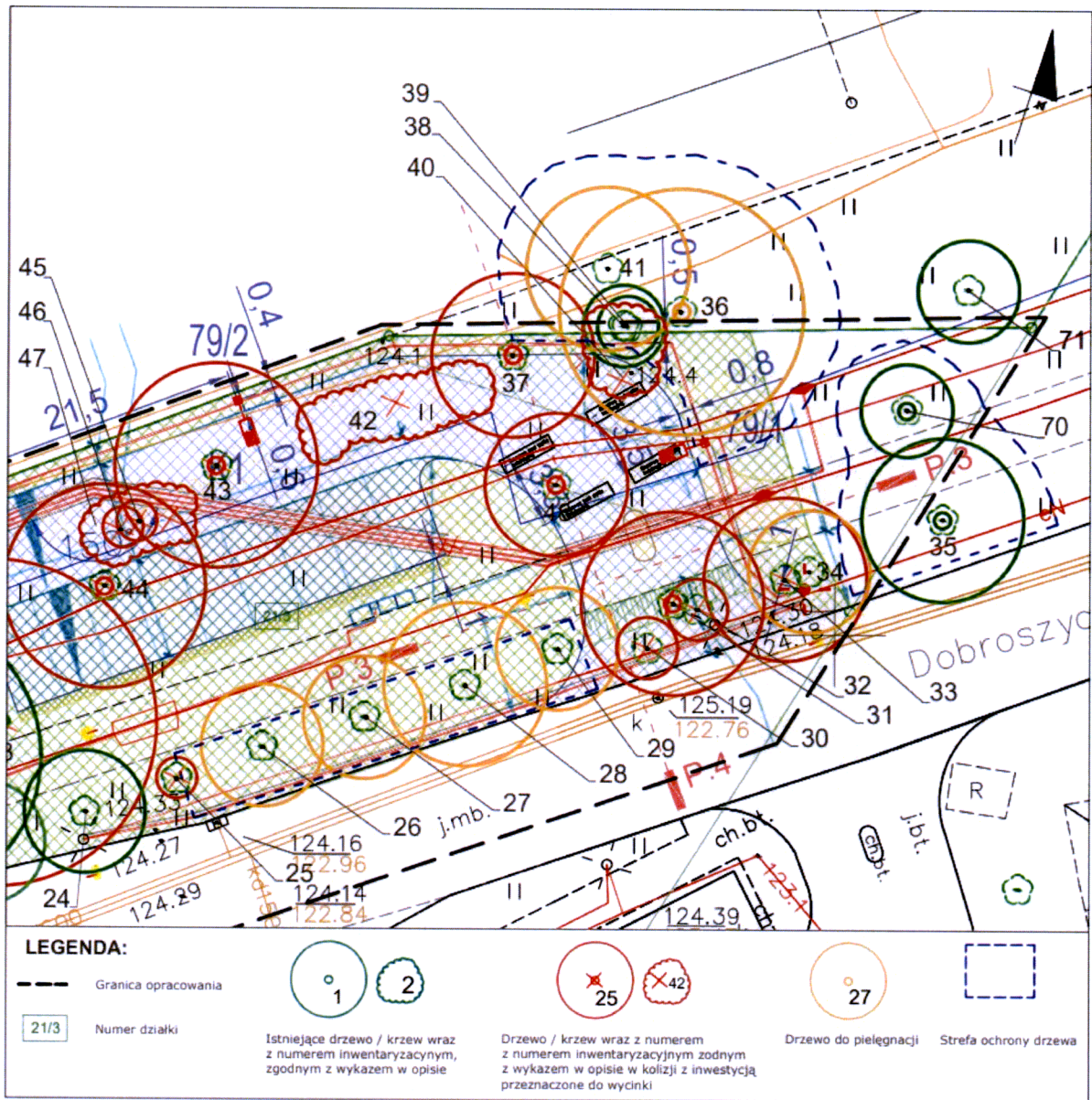
Ryc. 5. Przykładowy fragment rysunku operatu dendrologicznego na tle PZT (oprac. M. Kulon).
